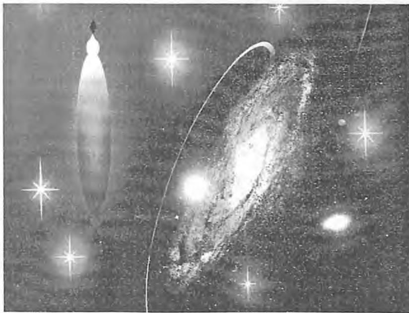
Туманность Андромеды
